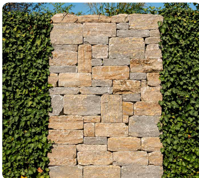
Muschelkalk Systemmauersteine, 14.5, 14.6, 14.7 (siehe Seite 5)
