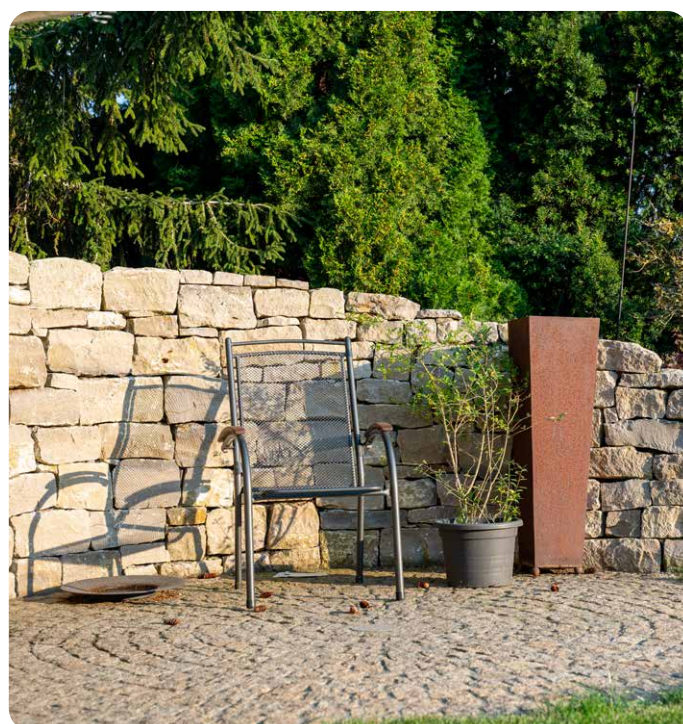
Trockenmauersteine Taubertal Kalkstein, TM5, TM6
