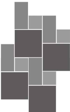
Verlegemuster für die Basalt Pflasterplatten PP007_A5 - PP007_F6
